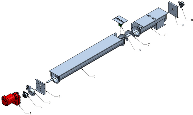
Abbildung 1: Trogförderschnecke Details
