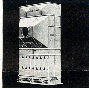
Durchlauftrockner MZ mit Stundenleistungen bis 100 t für Getreide, Mais etc.
