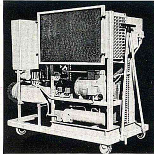
Kühlergeräte zur Konservierung von Getreide usw. Für Tagesleistungen von 25, 50, 100, 200 und 400 t
