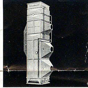
Radiatorentrockner mit Stundenleistungen bis 100 t für Getreide, Mais etc.
